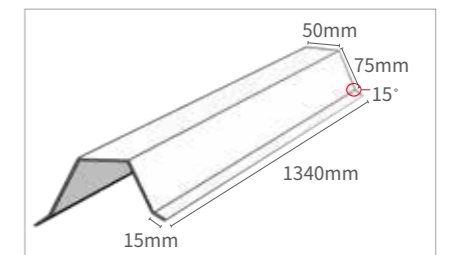
용마루 15 x 75 x 50 x 75 x 15 mm
